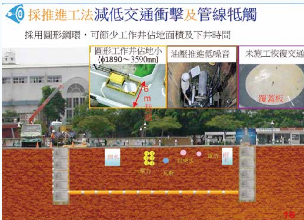
▲ 污水下水道工程採推進工法。
