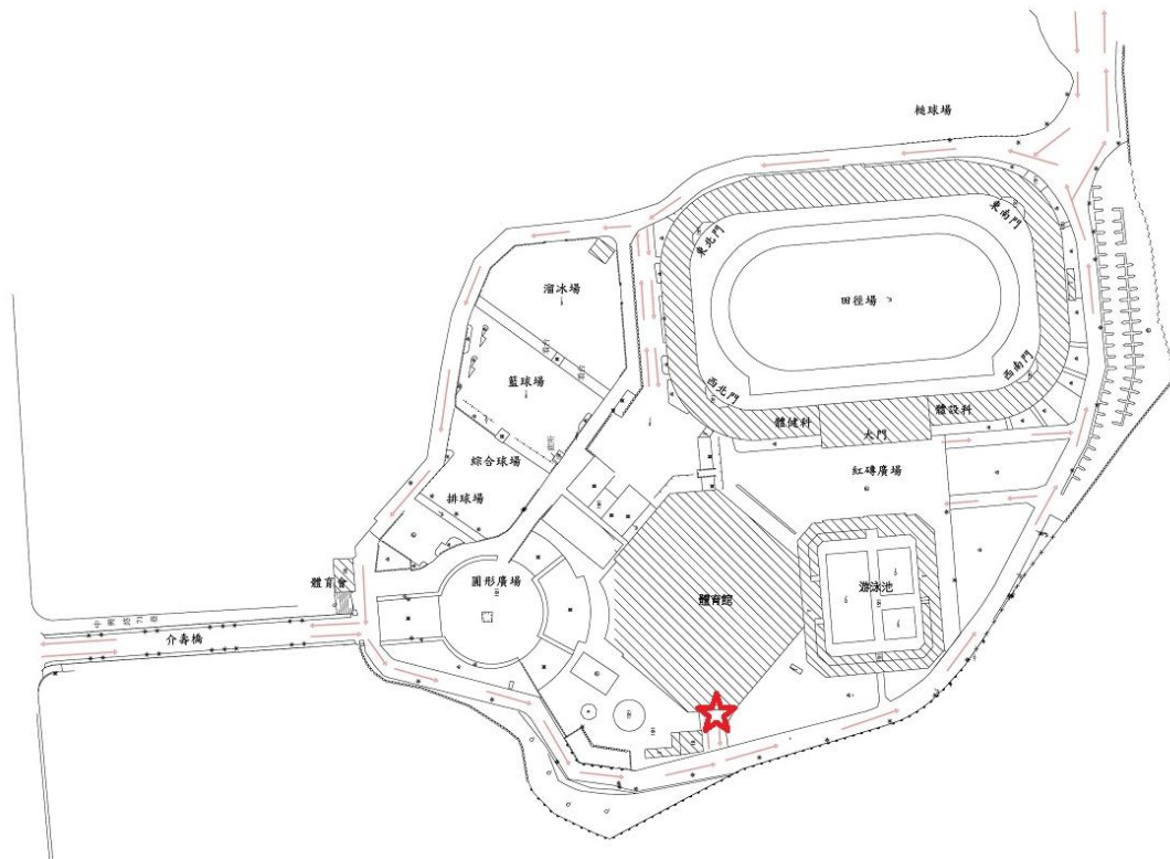
全區配置圖 S=1/2000
