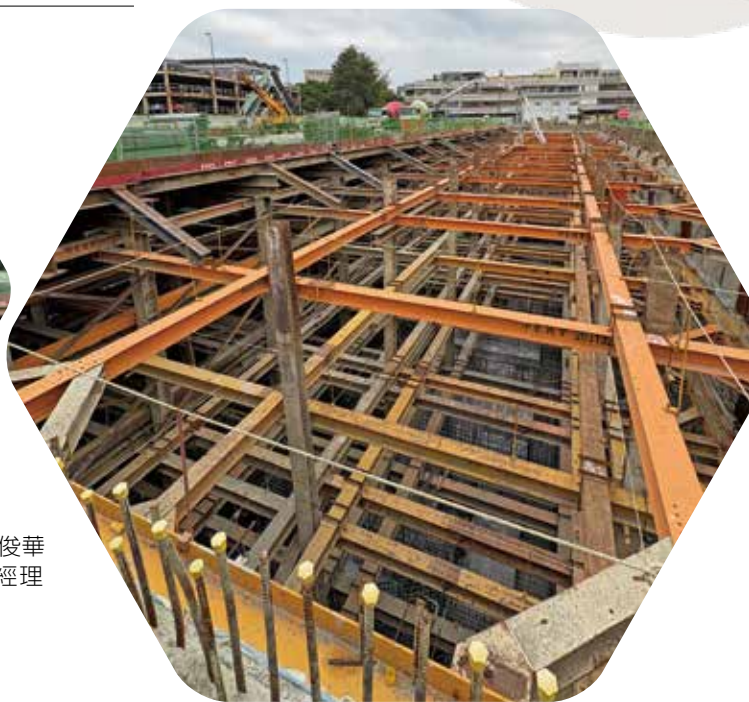
▲現場已完成混凝土大底澆置及地樑鋼筋綁紮、鋼模組立等工程，並正在進行筏基混凝土澆置。
